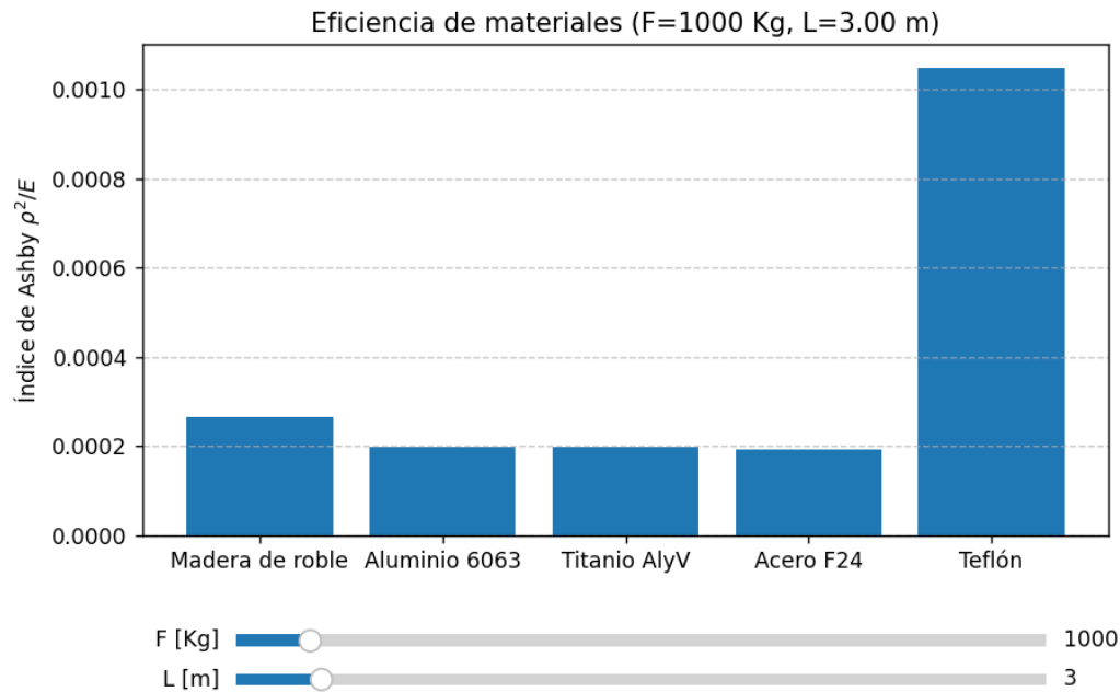
Figura 2: Eficiencia Rigidez / Peso de materiales.
